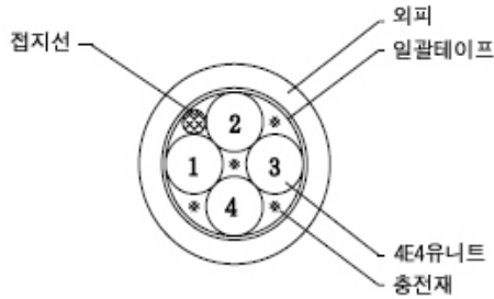
그림1. 구조도
