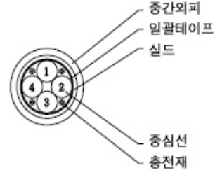
그림2. 4E4유니트 구조도
